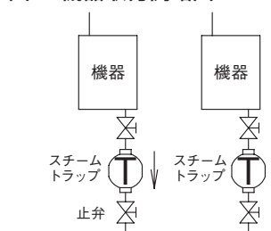
図8. 機器取付例略図
